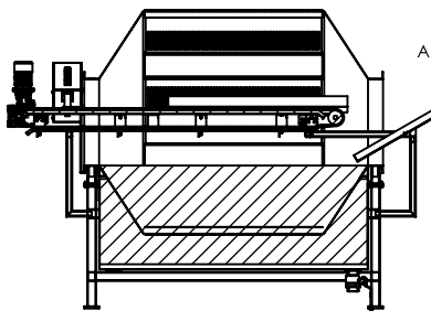
SECCIÓN A-A
